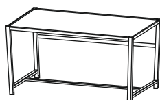
СИ-61 502.006 Габариты (д/ш/в): 1700x650x850 мм
